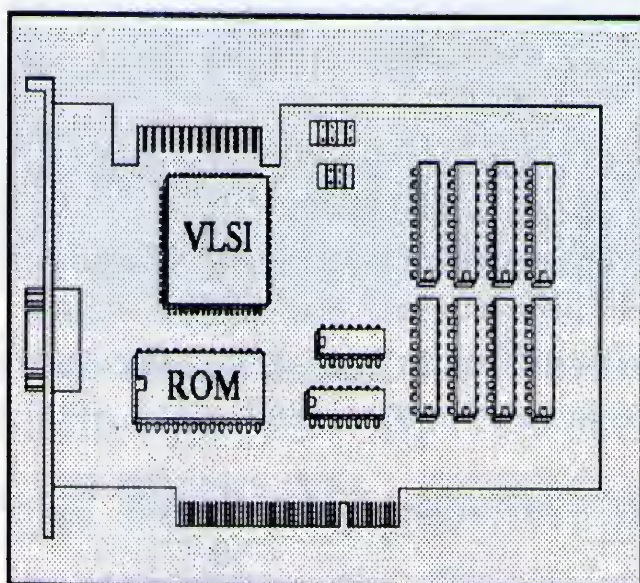
Figura 13 - placa SVGA de 64 bits (PCI)
